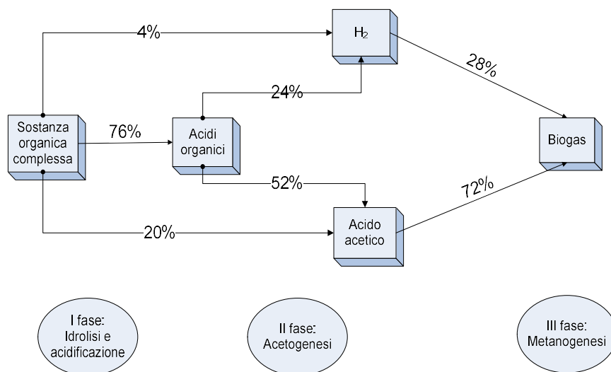
Fig. 3. Diagramma delle fasi di digestione anaerobica
