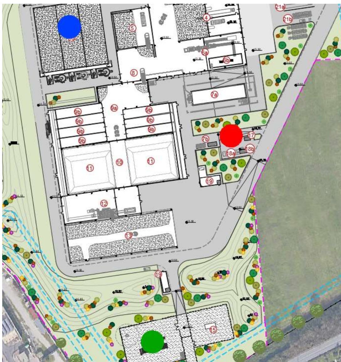
Fig.15.: Localizzazione delle sorgenti emmissive in progetto (in blu il biofiltro, in rosso la caldaia, in verde l'off-gas)
