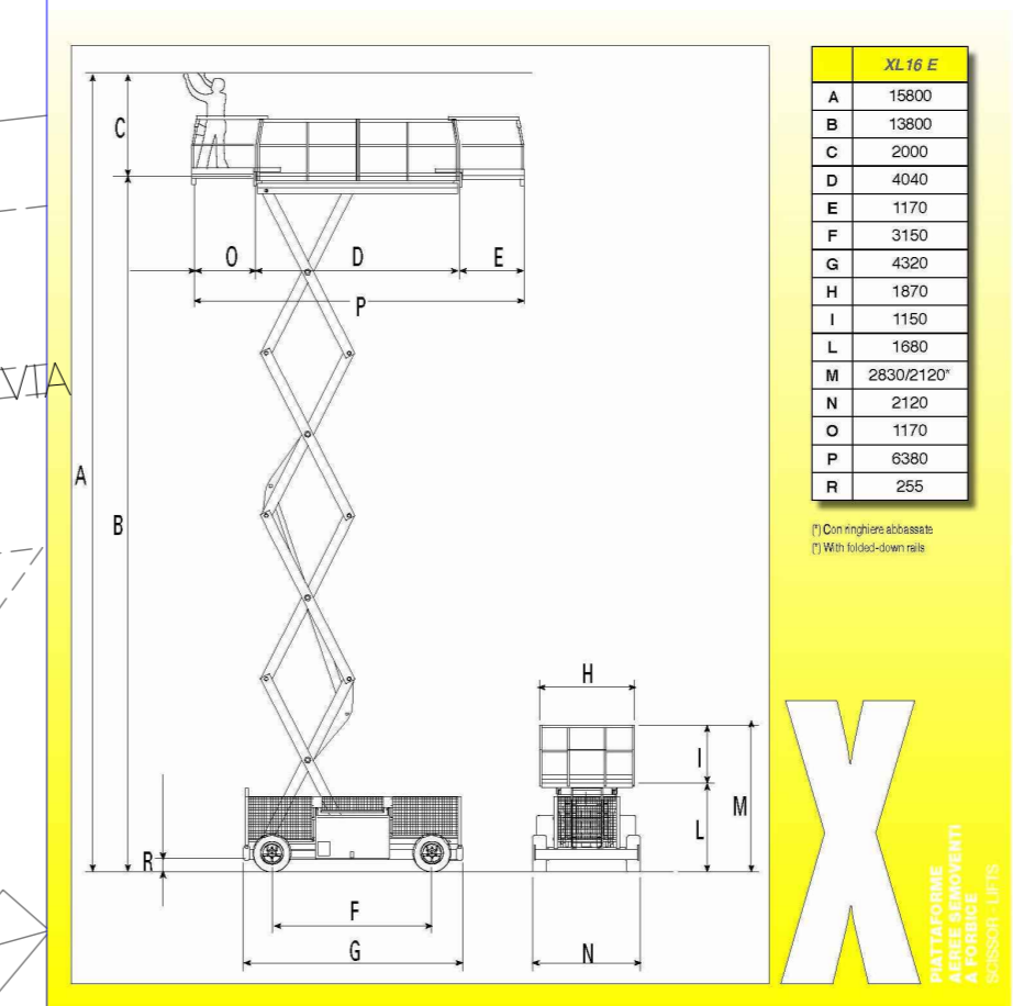
PIATTAFORMA PER ESTERNO TIPO
