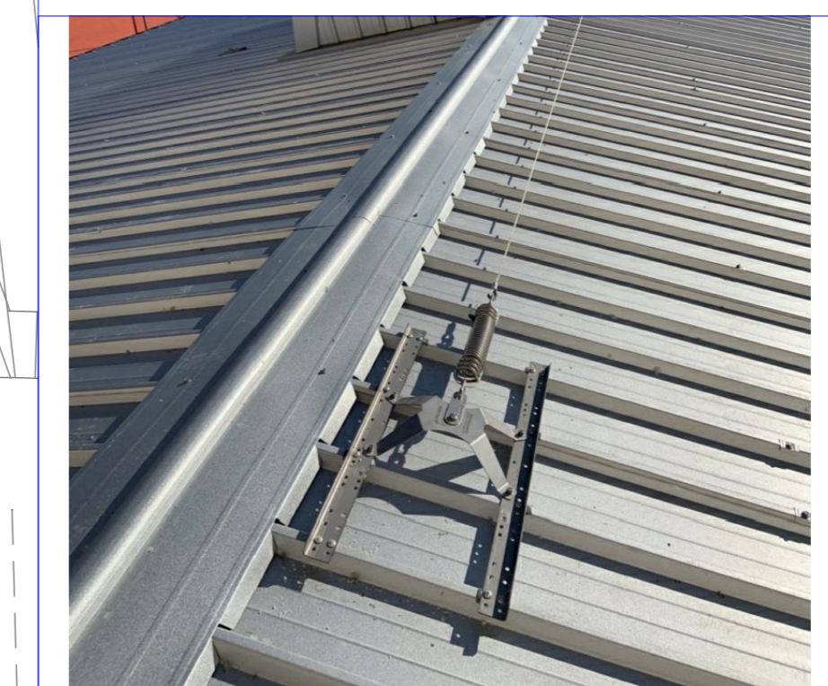
PIATTAFORMA PER ESTERNO TIPO
