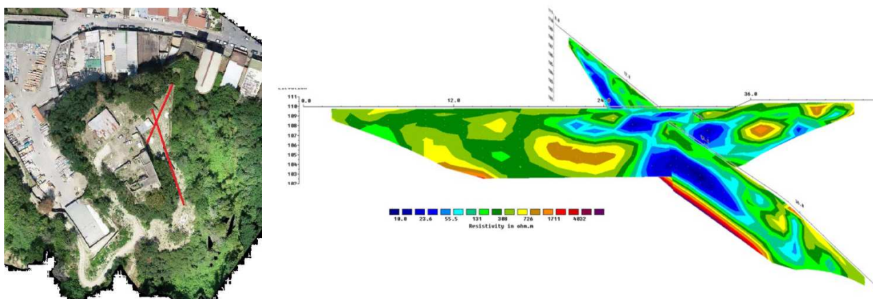
Figura 8. Ubicazione delle prospezioni geoelettriche nell'area in sommità alla cavità (a sinistra) e visualizzazione tridimensionale dei valori di resistività.
