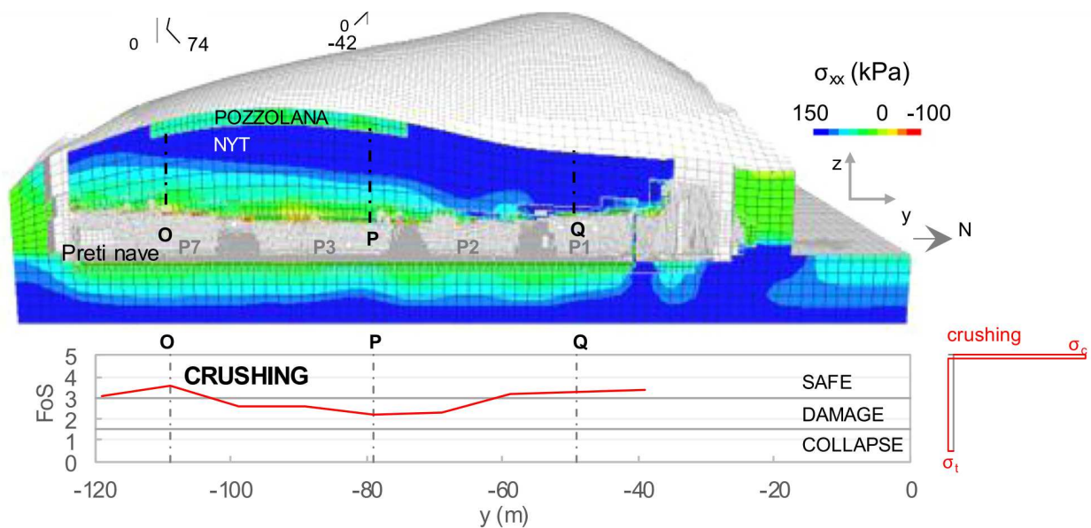
Figura 30. Tensioni orizzontali agenti e verifica della volta lungo la sezione passante per la “Navata dei Preti”.
