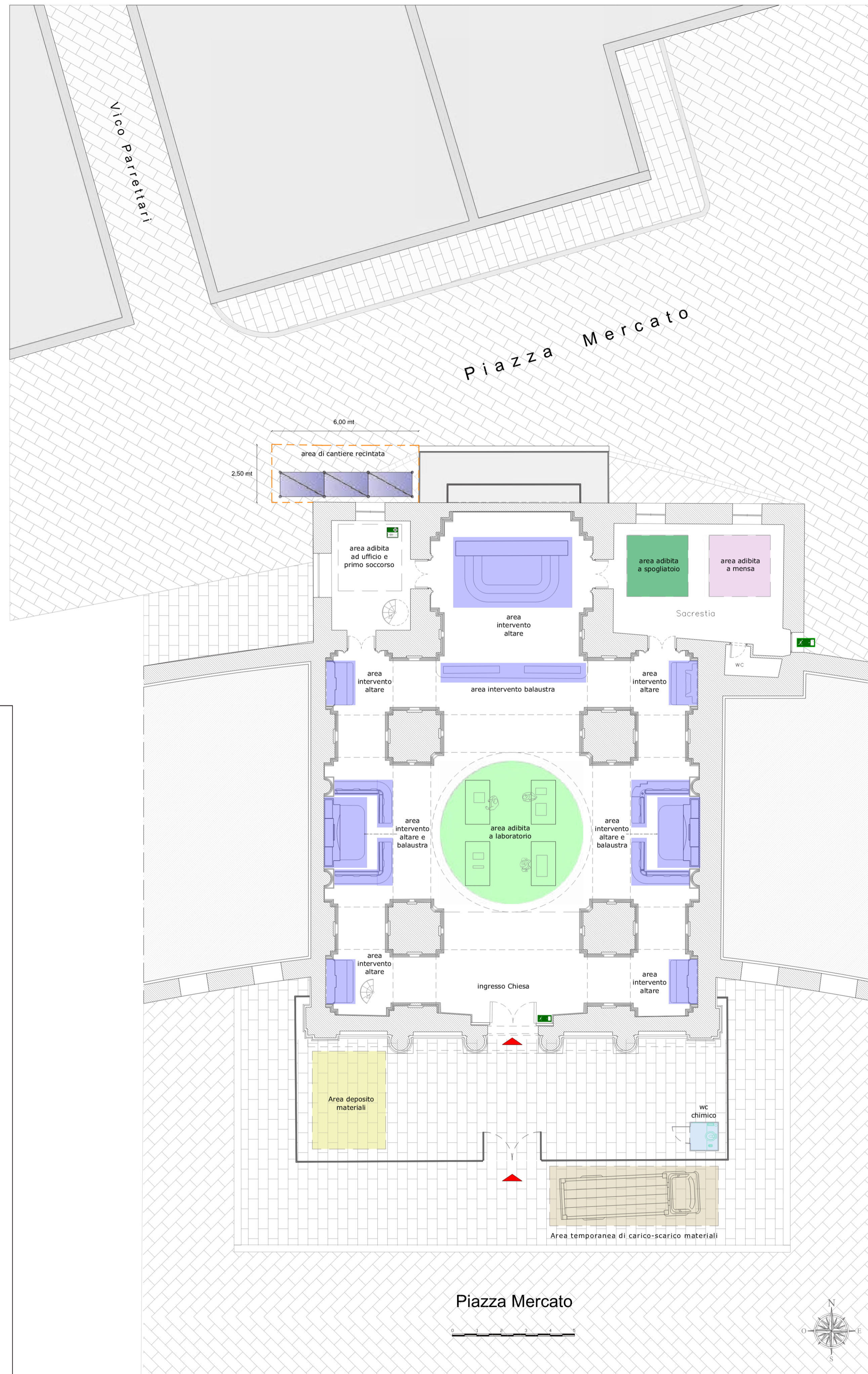
Planimetria LAYOUT DI CANTIERE
