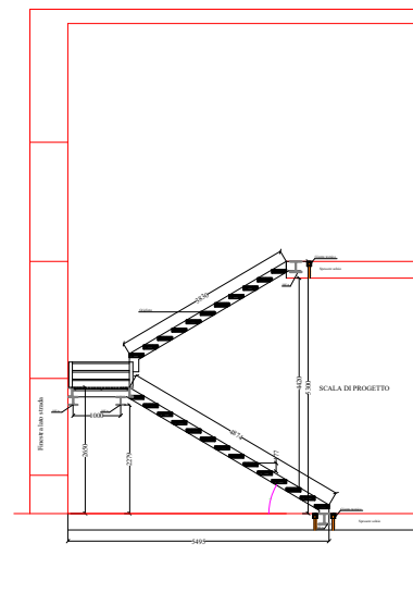
Sezione vano scala
