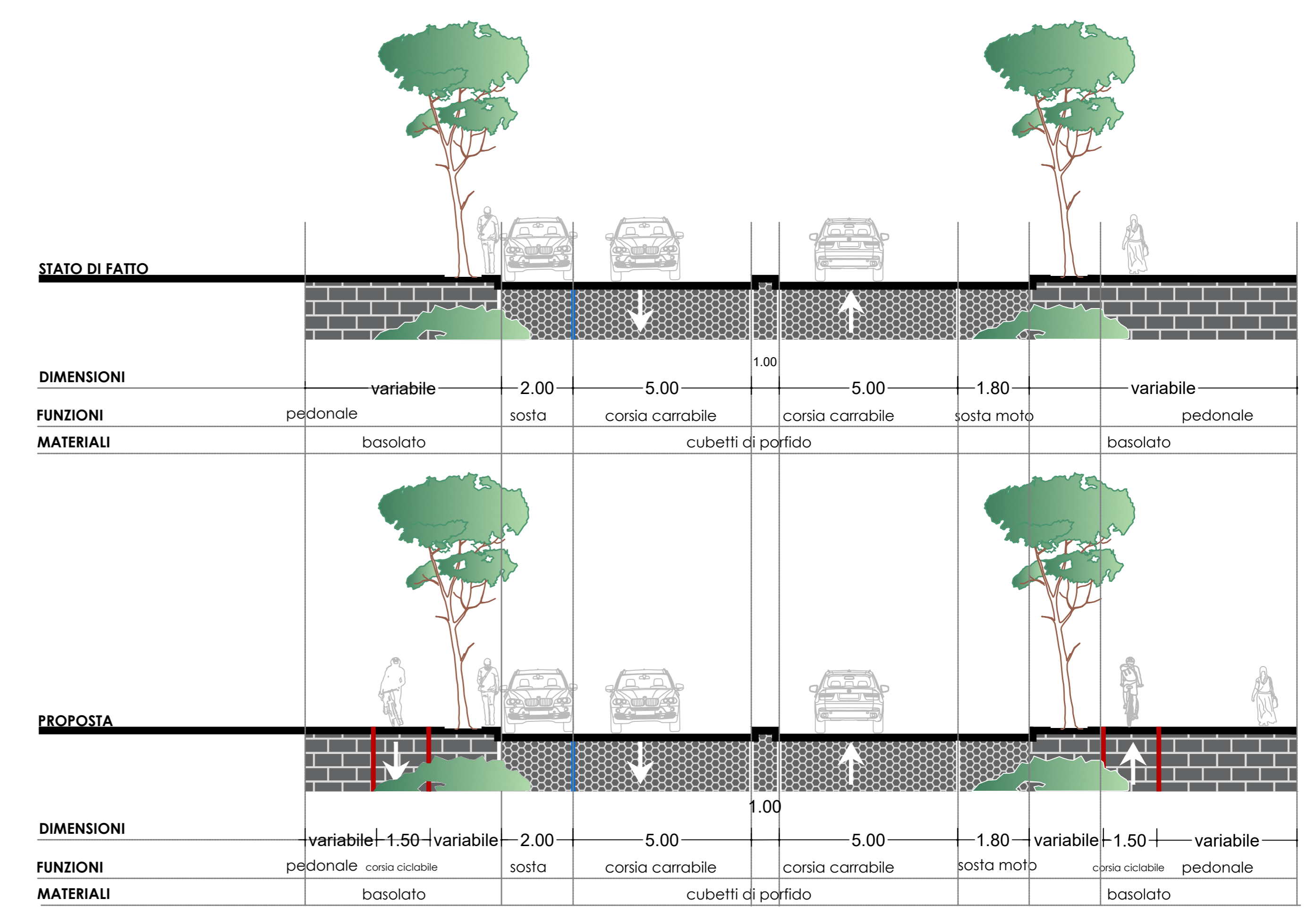
Via Foria Corsia ciclabile monodirezionale 1,50 m delineata a mezzo segnaletica su marciapiede
