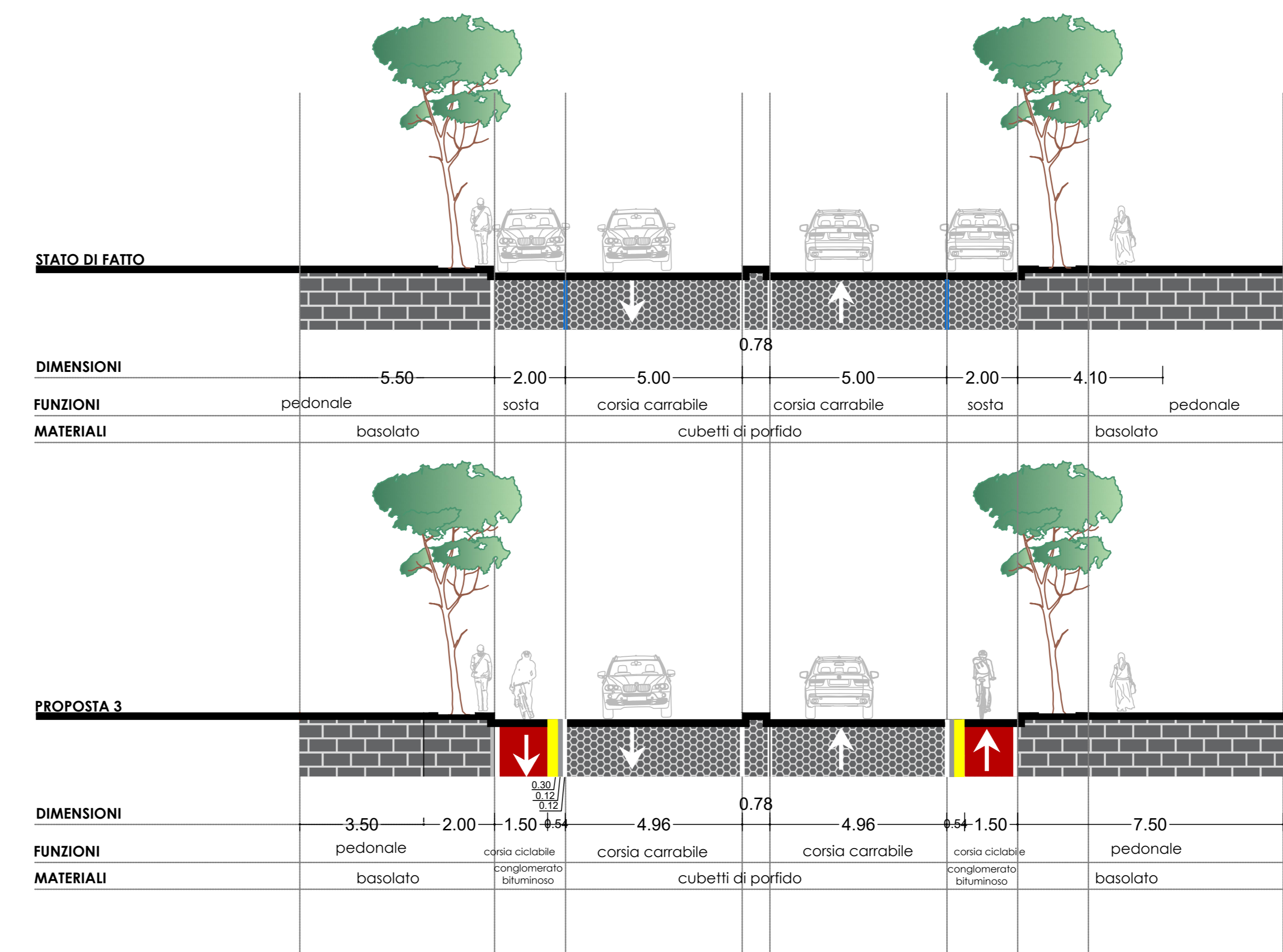
Via Foria Pista ciclabile monodirezionale di 1,50 m
