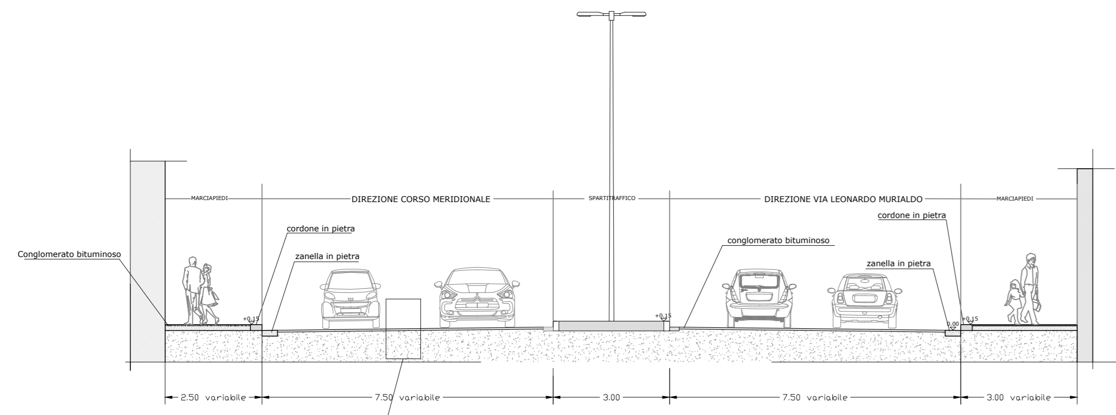
Scala 1:100
