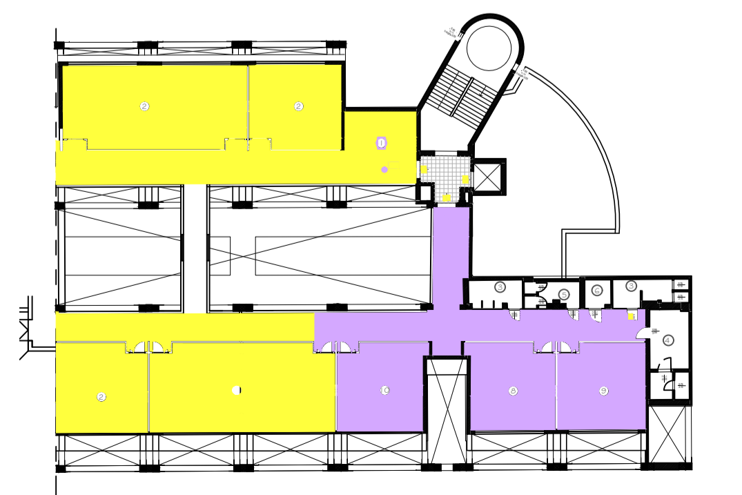
COMPARTIMENTI ANTINCENDIO PIANTA PIANO SECONDO
