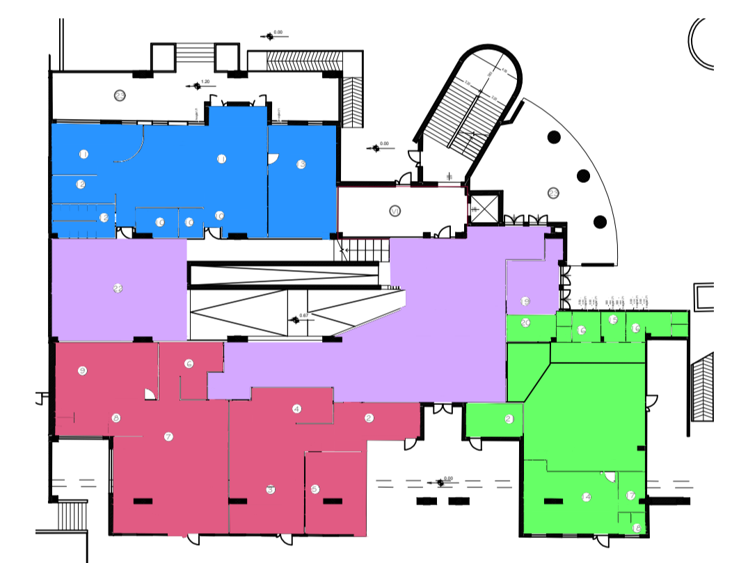
COMPARTIMENTI ANTINCENDIO PIANTA PIANO TERRA
