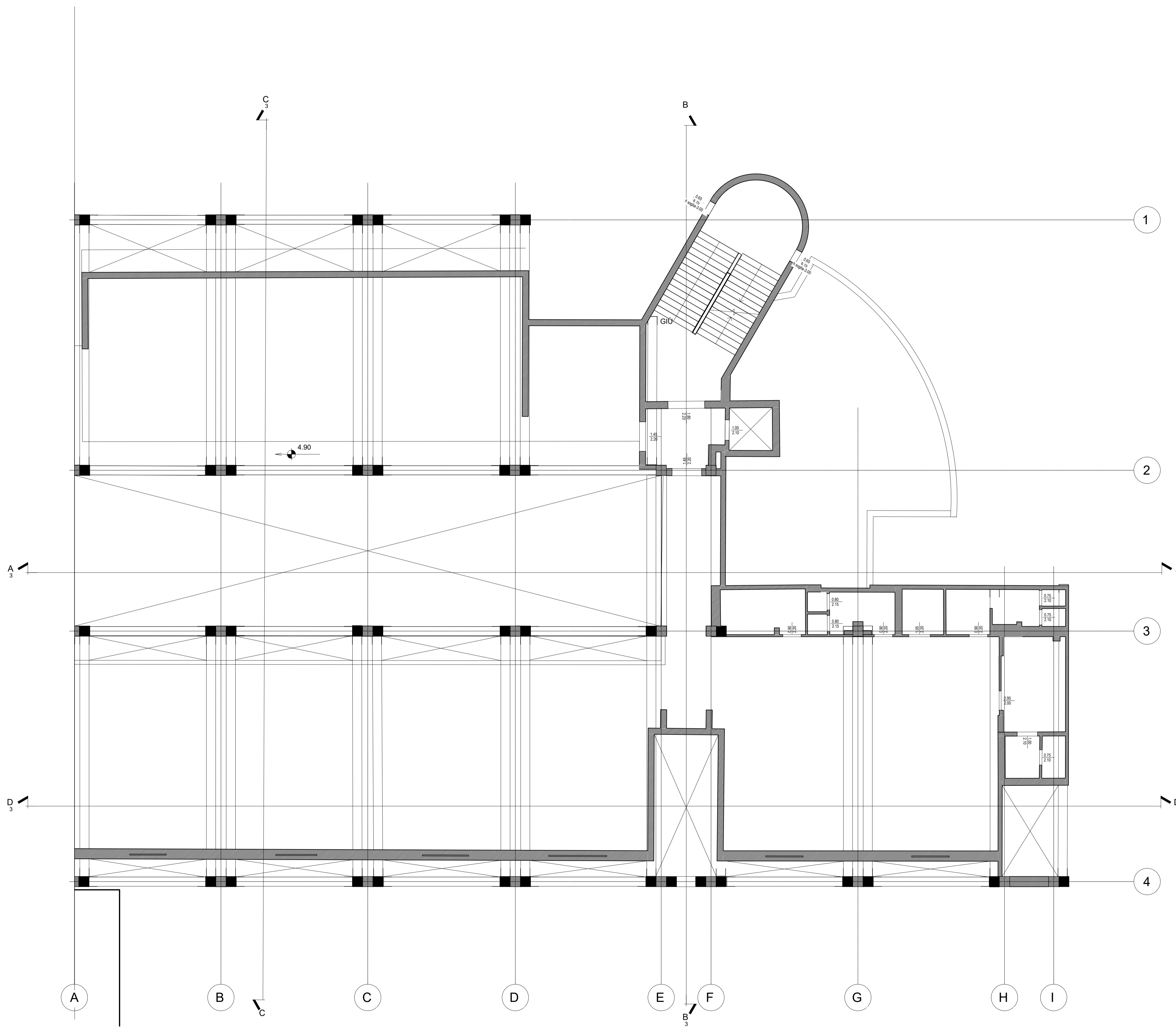
PIANTA PIANO PRIMO
