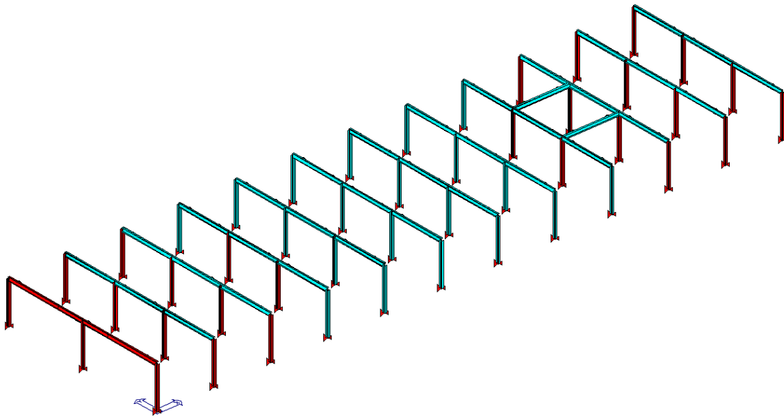
Figura 36 - Color Map membrature in acciaio. ag/g=80\%
