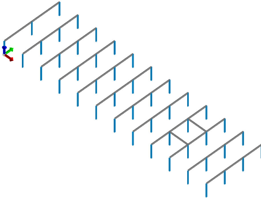
Figura 29 - Vista Posteriore prospettica modello strutturale
