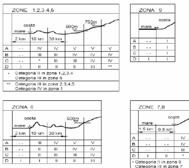
Figura 17- Definizione delle categorie di esposizione
