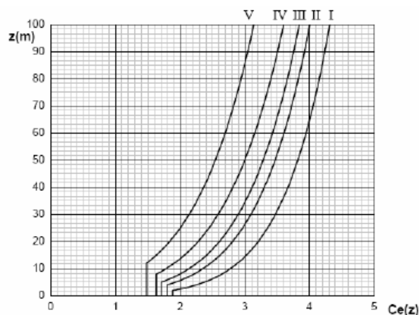
Figura 19 - Andamento del coefficiente di esposizione c_e in funzione dell'altezza sul suolo (per c_t=1 )
