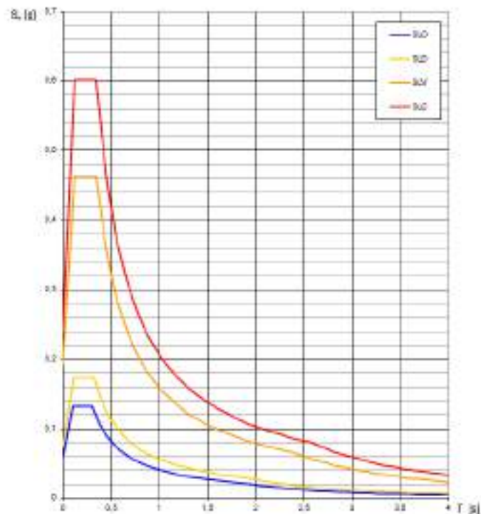
Figura 26 - Spettri elastici per i diversi stati limite
