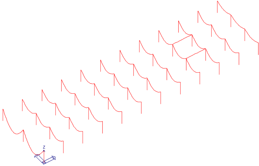
Figura 30 - Deformata SLU
