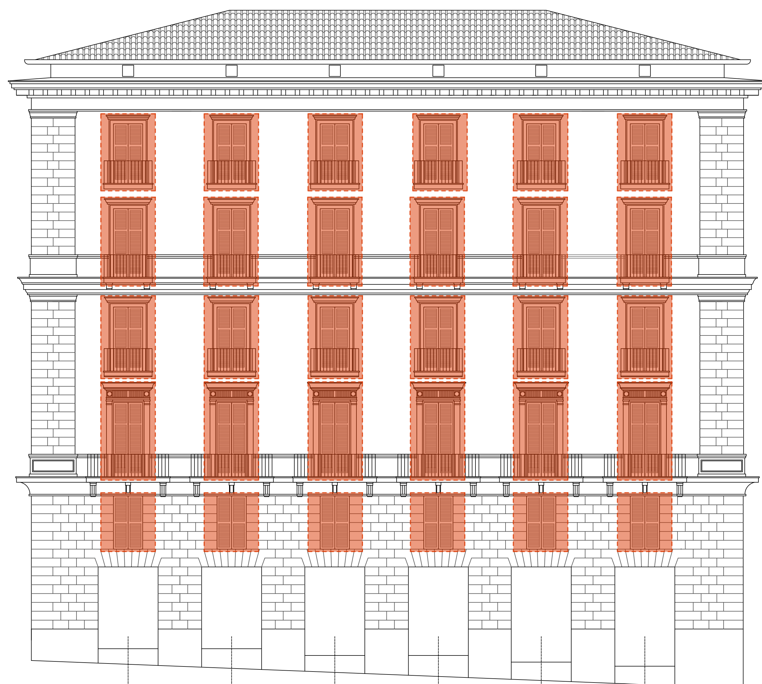
PROSPETTO A EST SU VIA LEONCAVALLO
