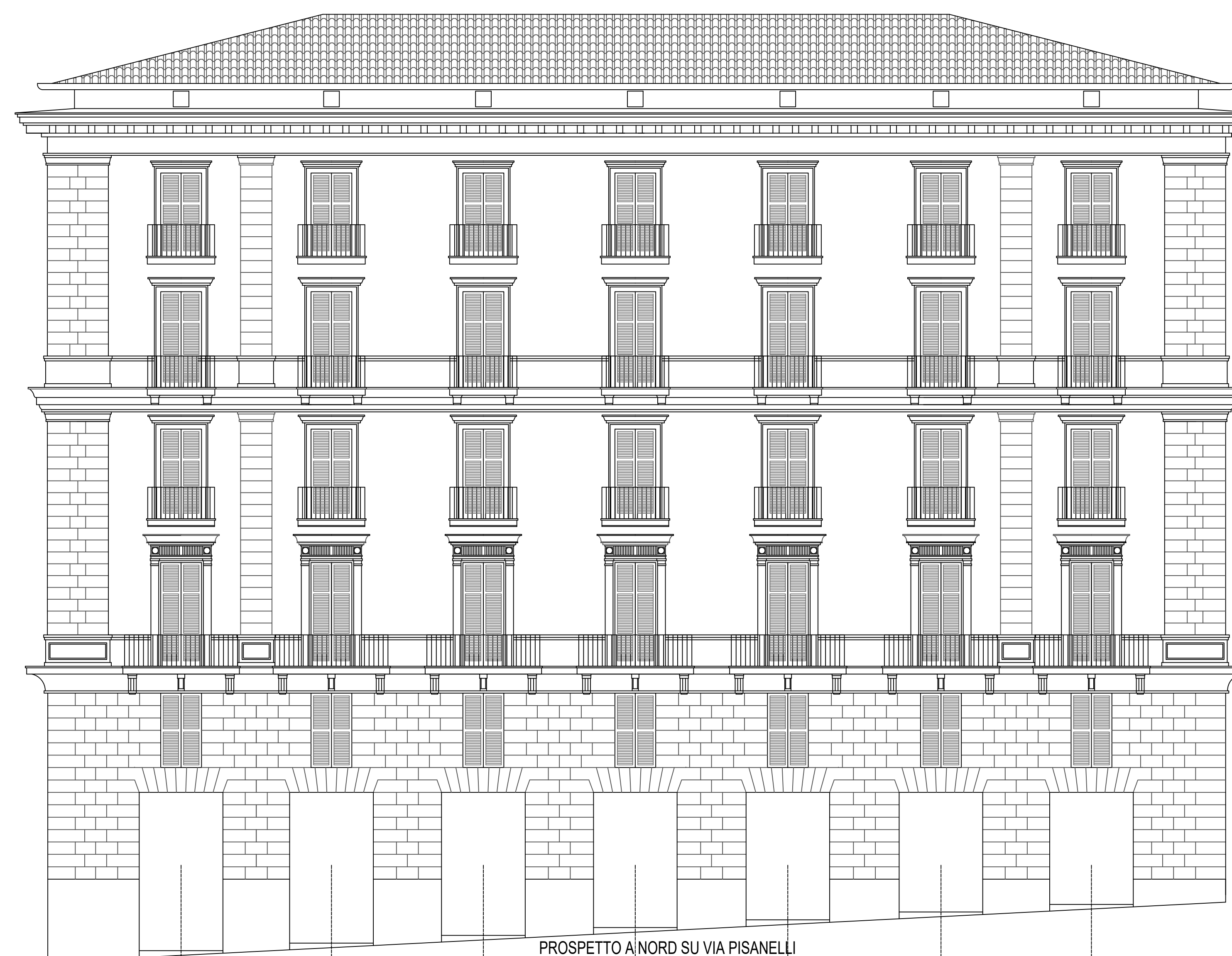
PROSPETTO A NORD SU VIA PISANELLI
