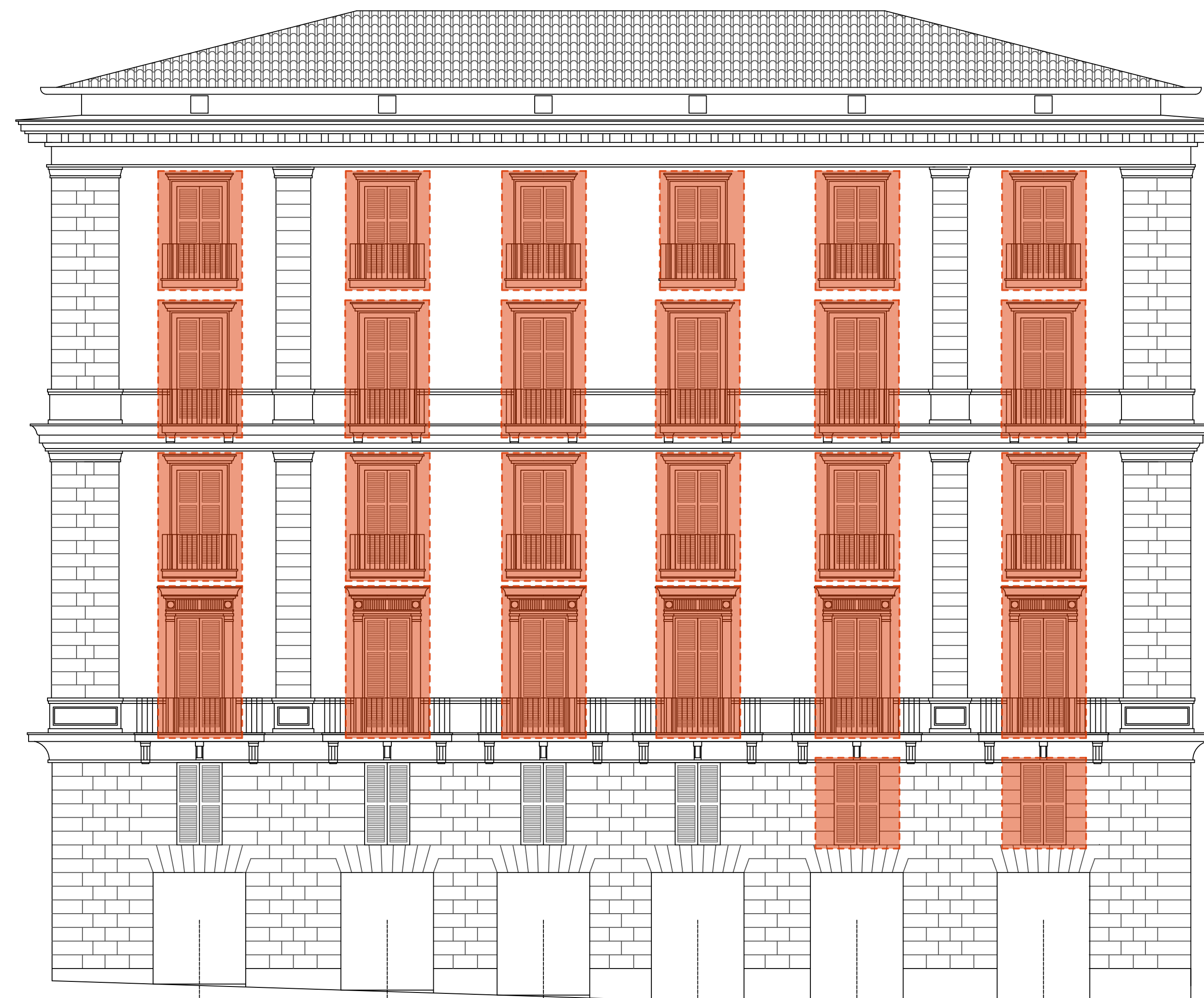
PROSPETTO A SUD SU VIA SANTA BRIGIDA
