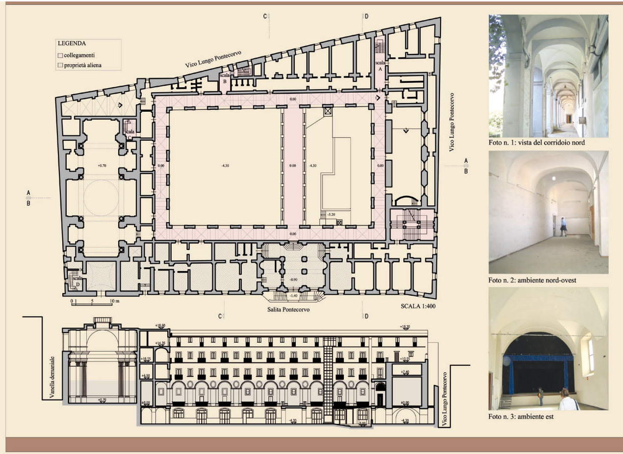
Rilievo Pianta piano primo – Sezione A-A'
