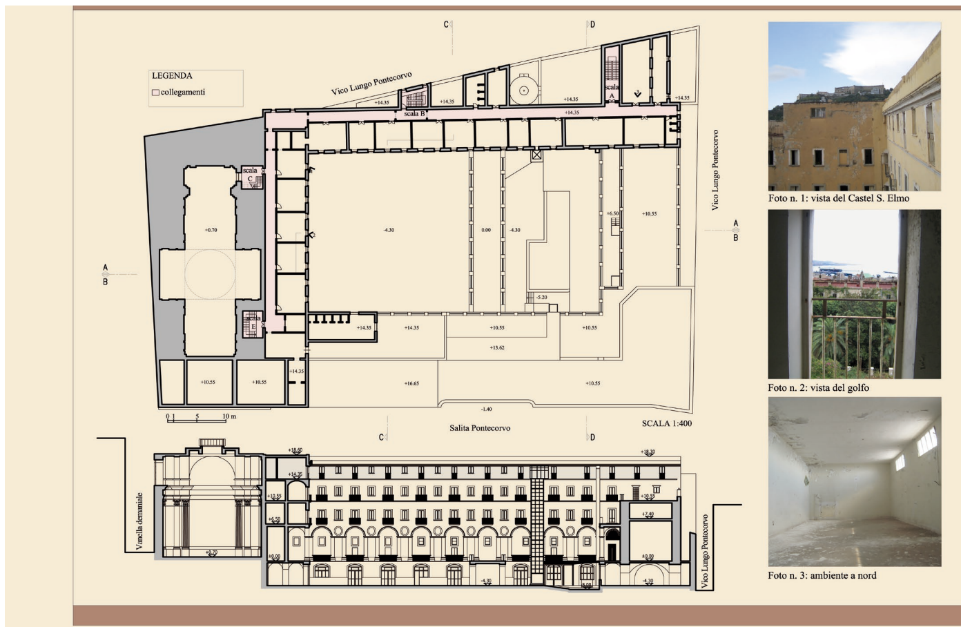
Rilievo Pianta piano quarto – Sezione A- A'
