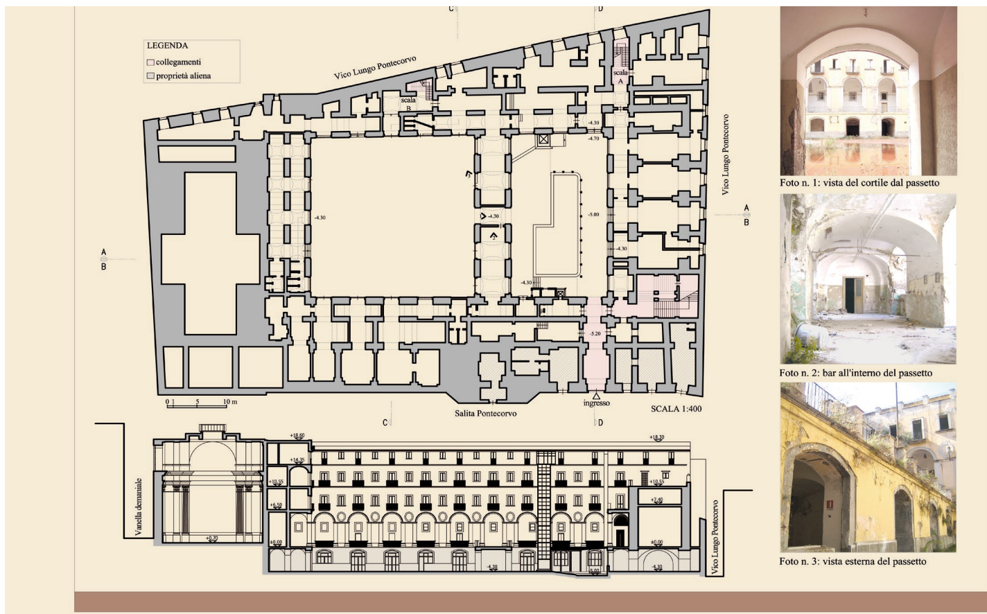
Rilievo Pianta piano terra – Sezione A- A'
