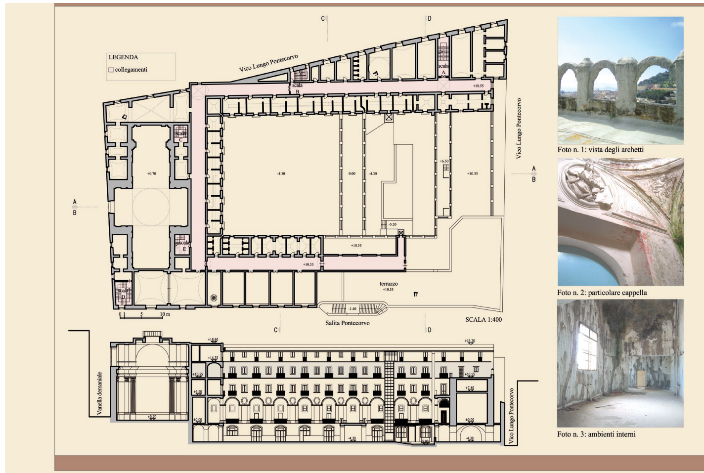
Rilievo Pianta piano terzo – Sezione A- A'
