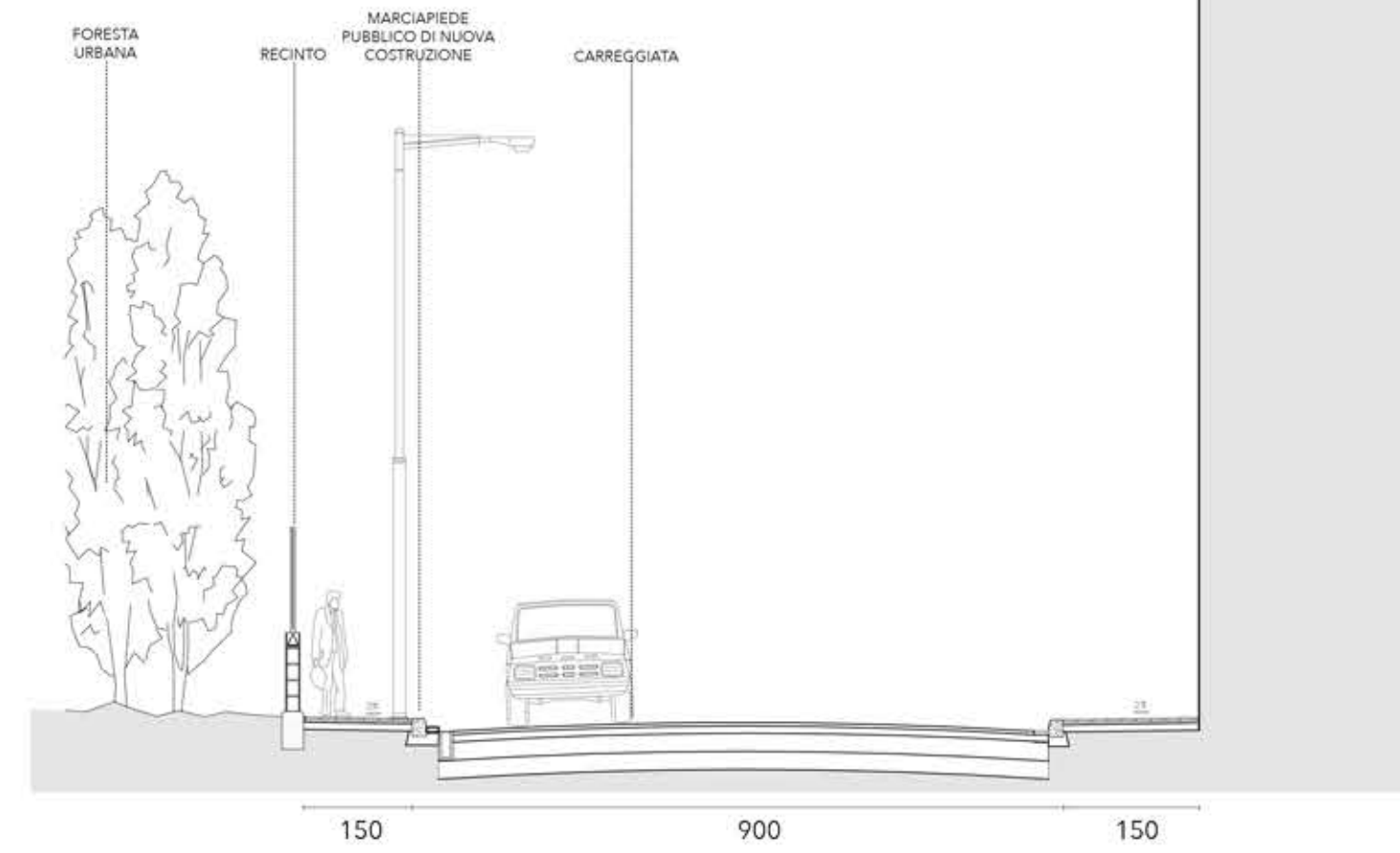
Sezione stradale_scala 1:100
