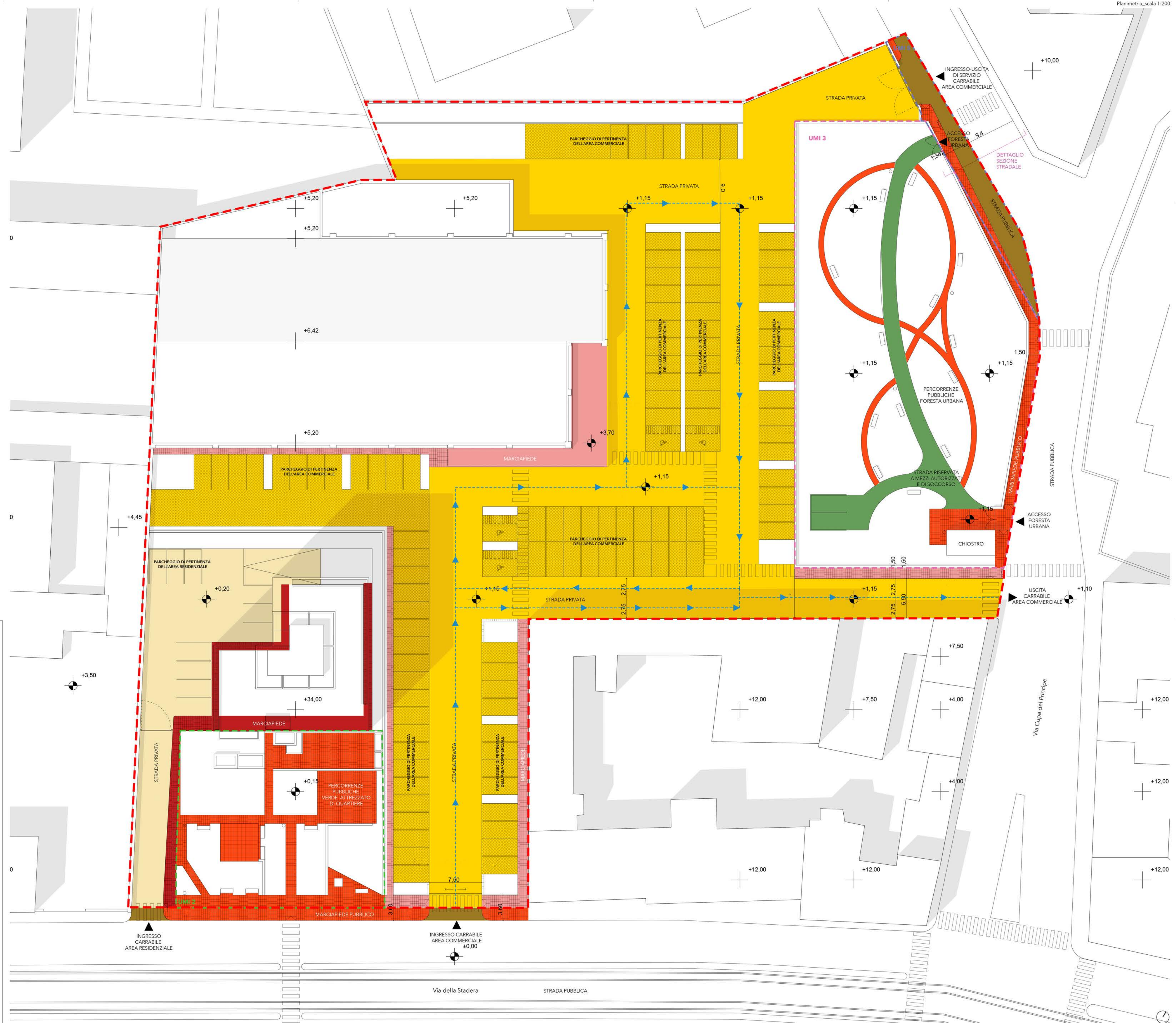
Planimetria_scala 1:200
