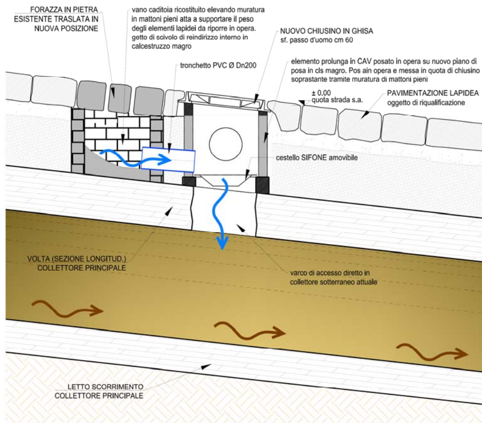
Figura 4 - soluzione spostamento caditoia storica a fessura e suo sifonamento
