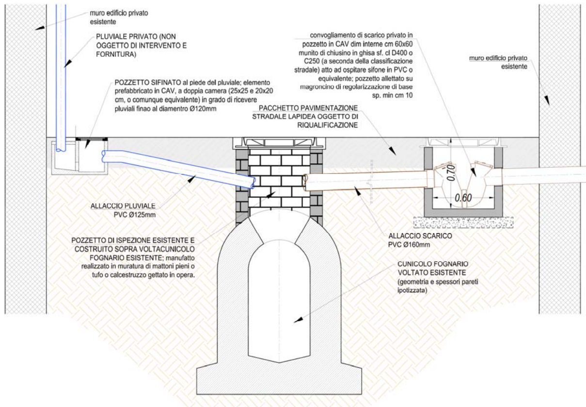
Figura 7 - schema riallaccio scarichi e pluviali
