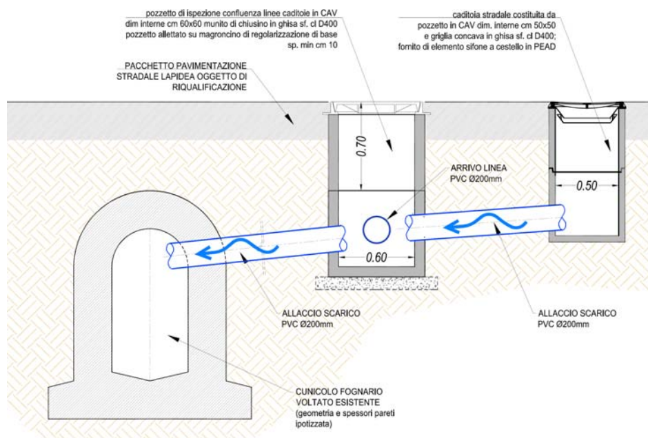
Figura 6 - schema allaccio caditoie NON in serie
