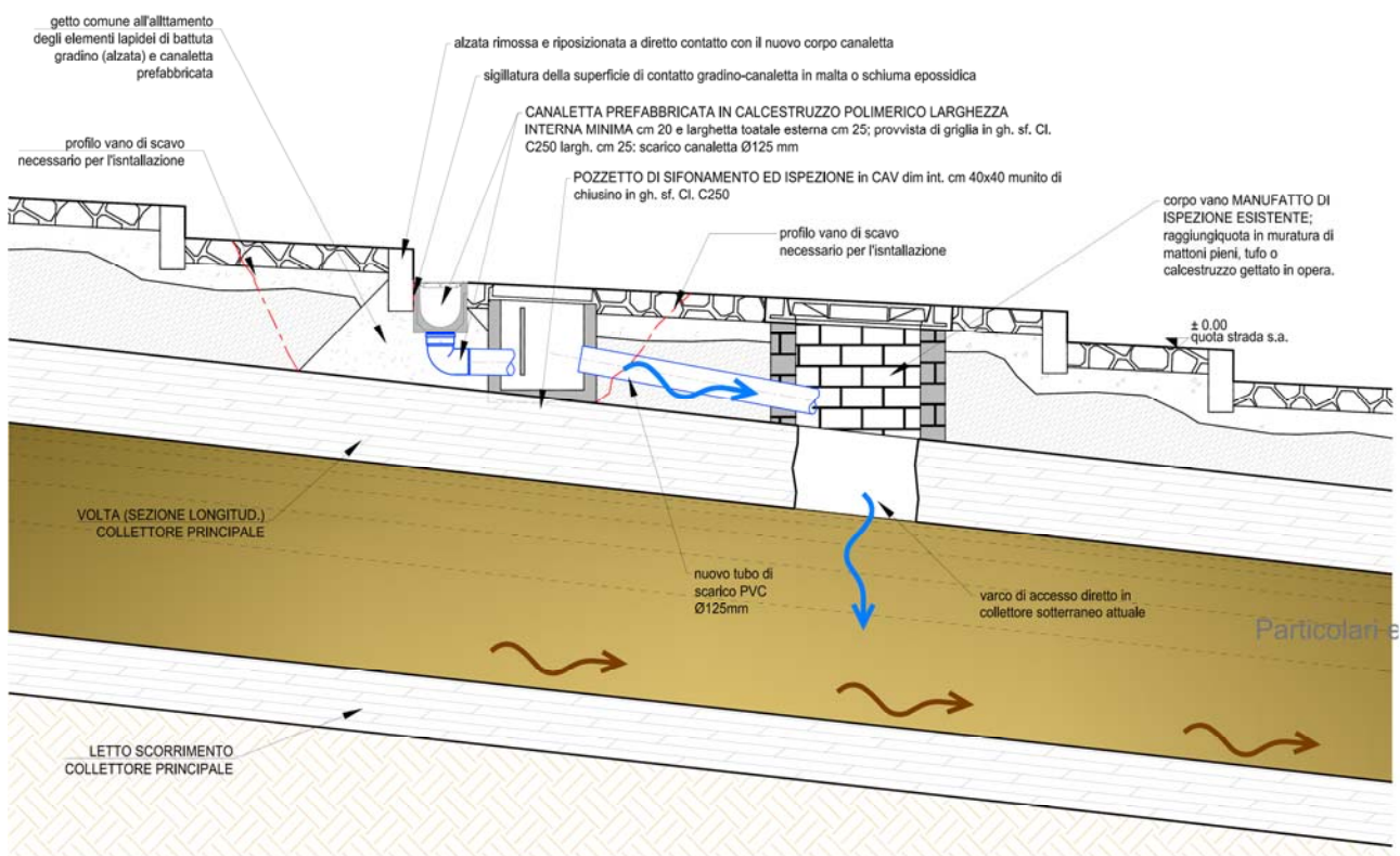
Figura 5 - inserimento di canalette a ridosso delle alzate gradinate esistenti
