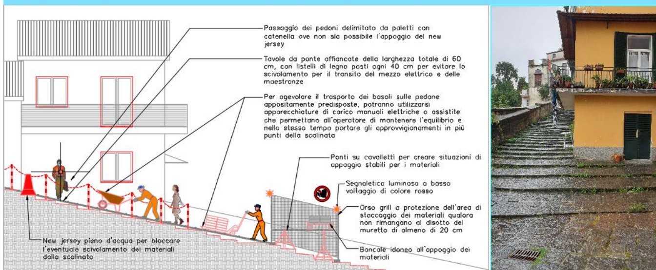
Tipologico delle lavorazioni lungo la scalinata
