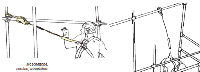
Ancoraggio puntuale per gli interventi di prelievo materiali dal ponteggio
