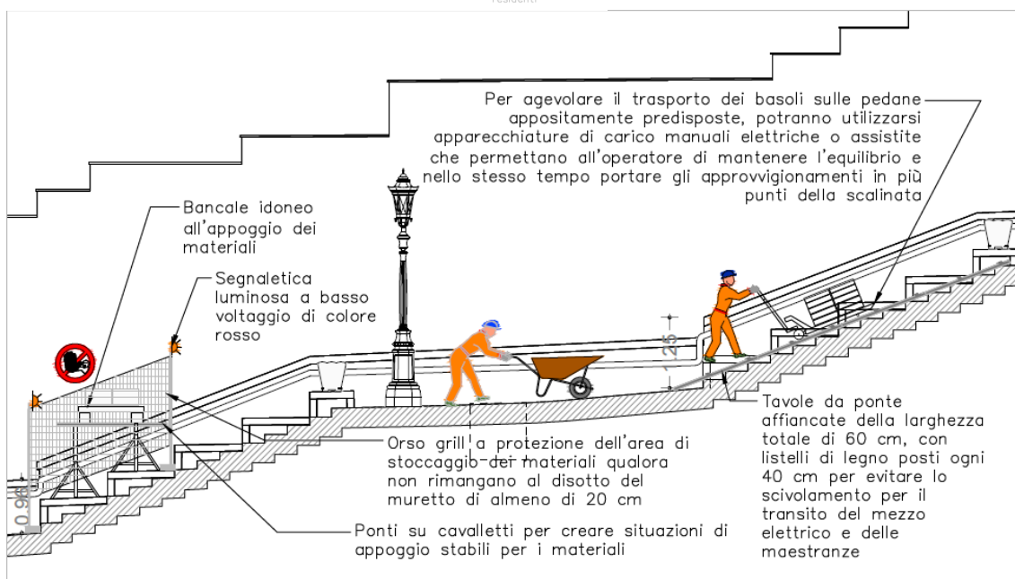
Tipologico delle lavorazioni lungo la scalinata
