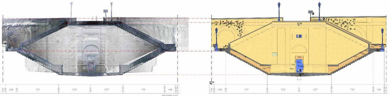
Figura 8 Stralcio elaborato Stato di Conservazione- serie CNAP001GKE- Scala monumentale di Montesanto – Sezione trasversale
