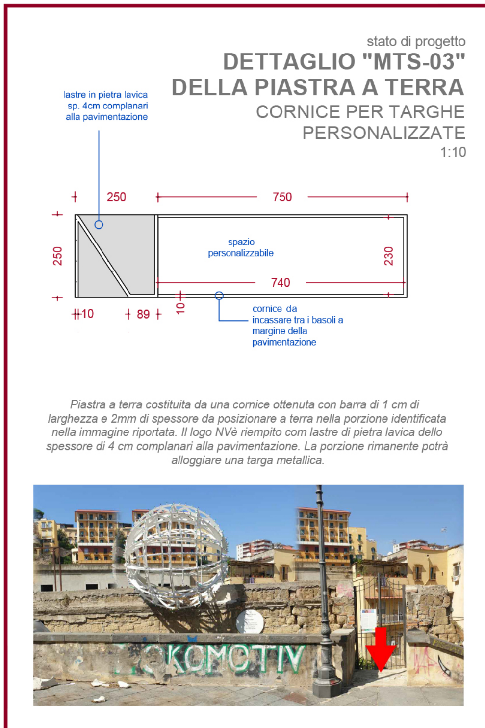
Figura 17 Tavola di progetto
