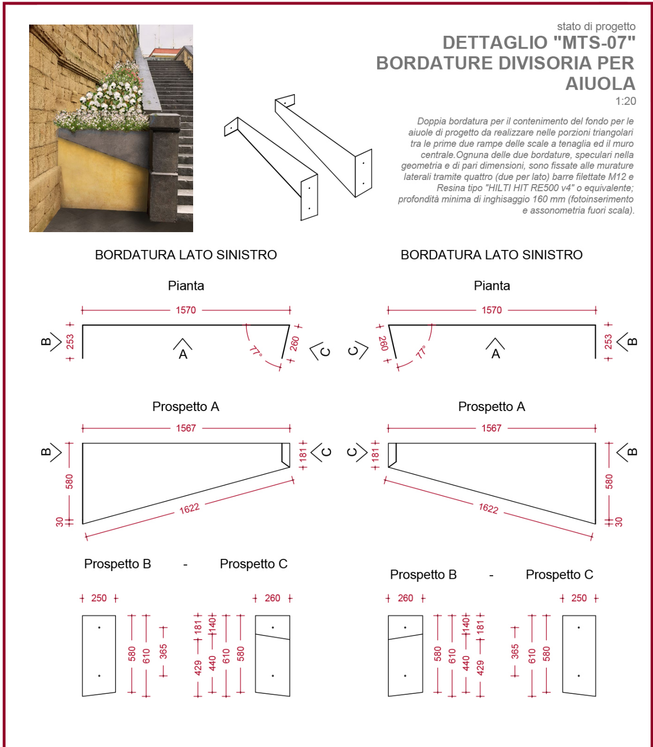
Figura 16 Tavola di progetto
