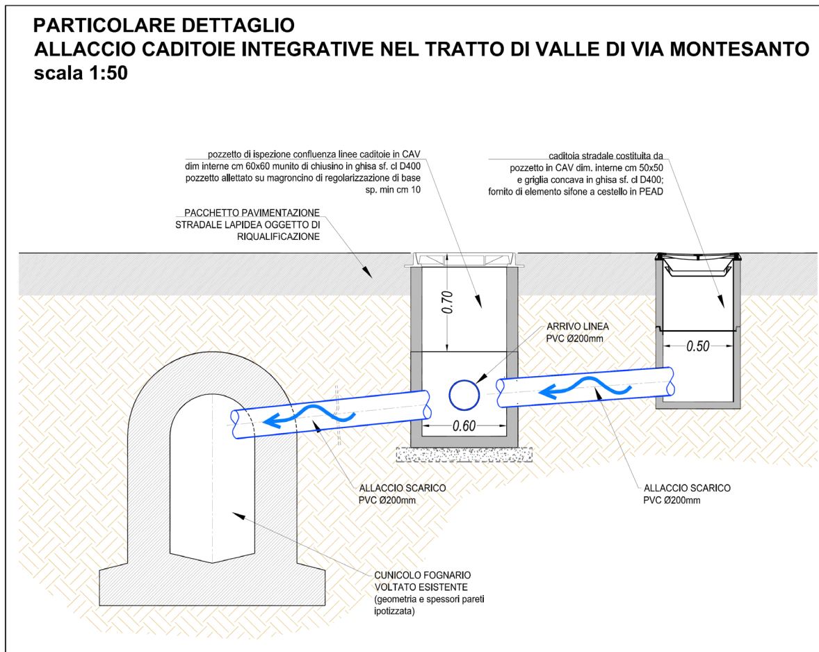
Figura 26 - estratto tavola grafica di progetto
