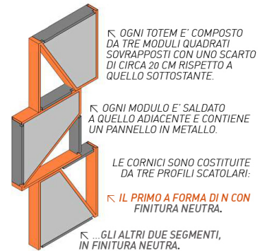
Figura 13_Totem – elaborato esecutivo
