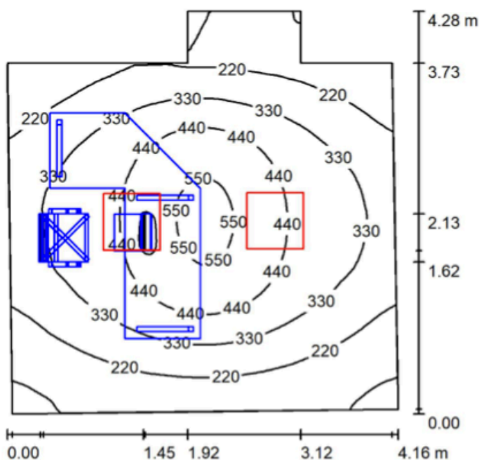
Altezza locale: 3.500 m, Altezza di montaggio: 3.200 m, Fattore di manutenzione: 0.80
