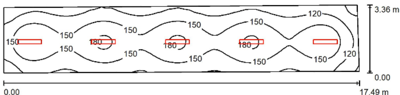
Altezza locale: 3.500 m, Altezza di montaggio: 3.500 m, Fattore di manutenzione: 0.80
