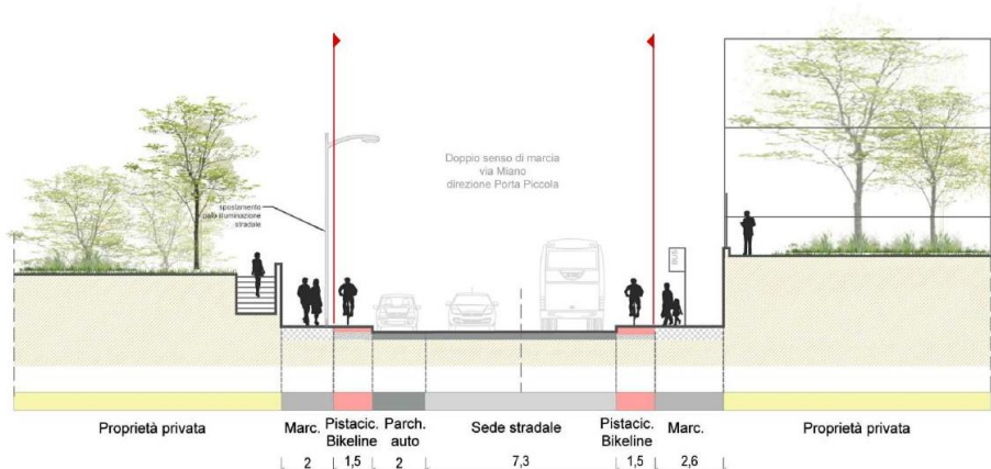
SEZIONE B-B' PROGETTO
