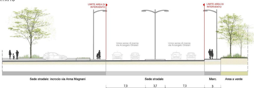
SEZIONE A-A' STATO DI FATTO
