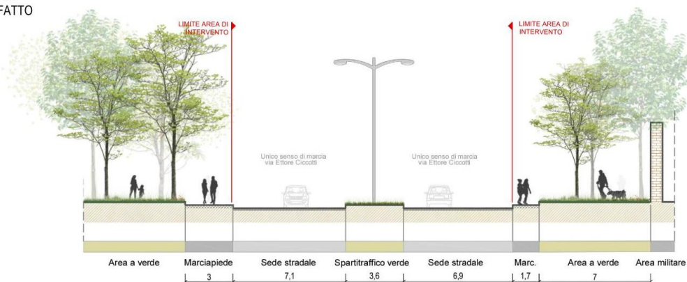
SEZIONE A-A' STATO DI FATTO
