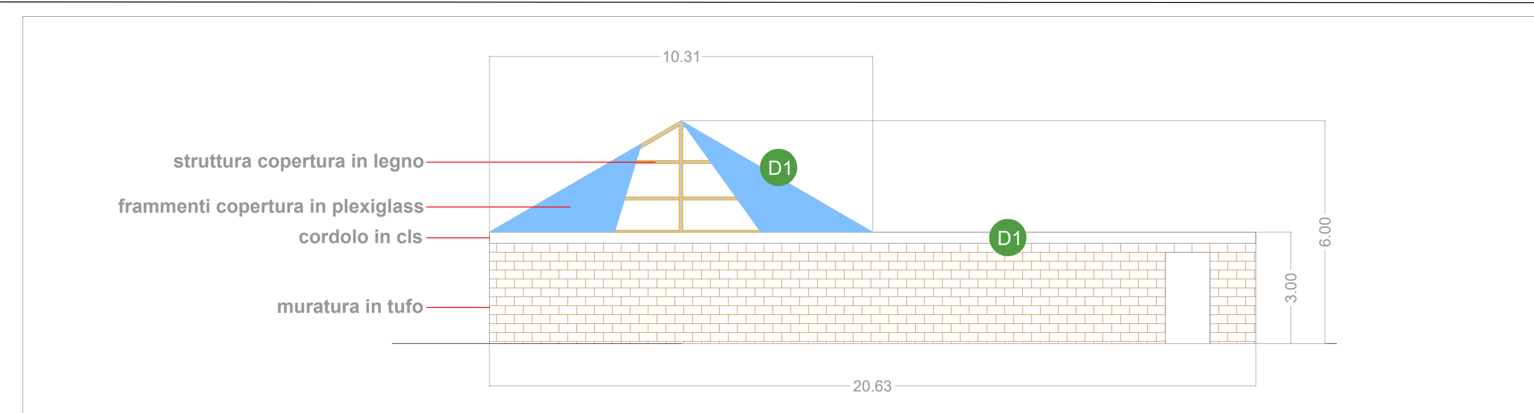
Prospetto frontale giardino d'inverno
