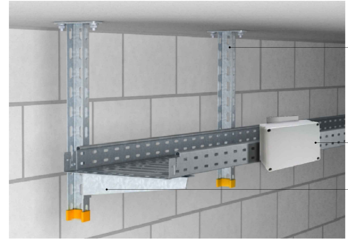
CANALINA E CASSETTA DI DERIVAZIONE
