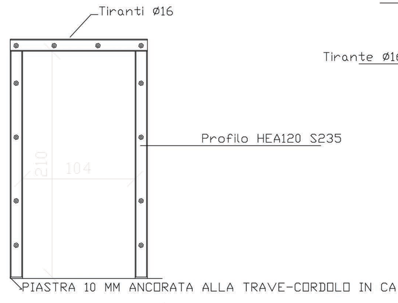
PARTICOLARE ANCORAGGIO TRAVE-CORDOLO IN CA
