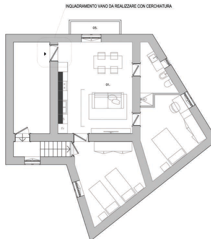
PIANTA SCALA 1:100 - STATO DI FATTO
