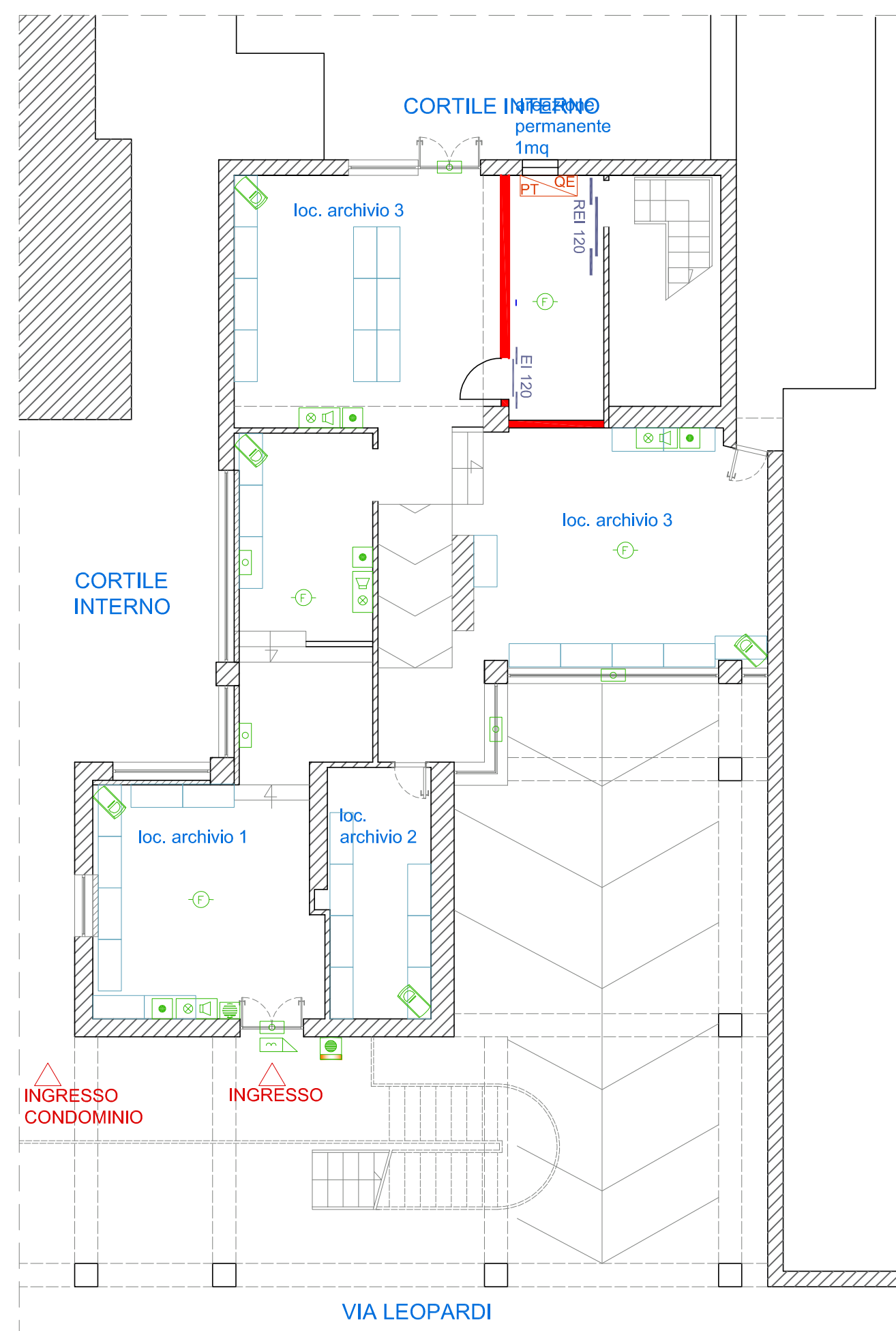
PIANTA PIANO TERRA ARCHIVIO 2
