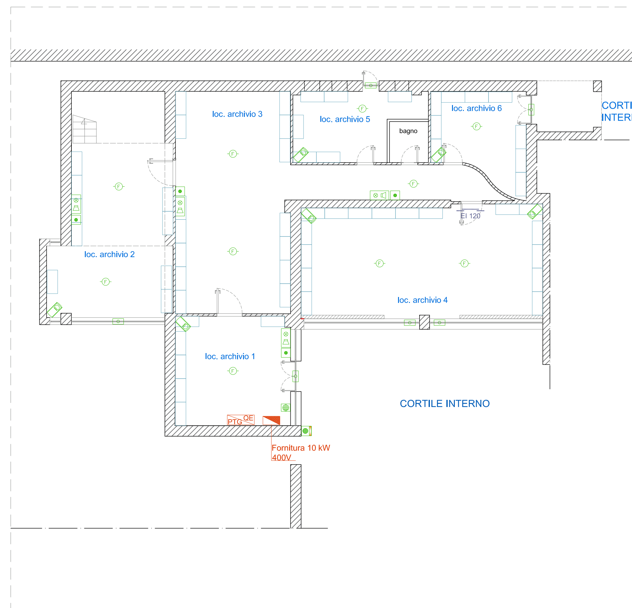
PIANTA PIANO TERRA ARCHIVIO 1
