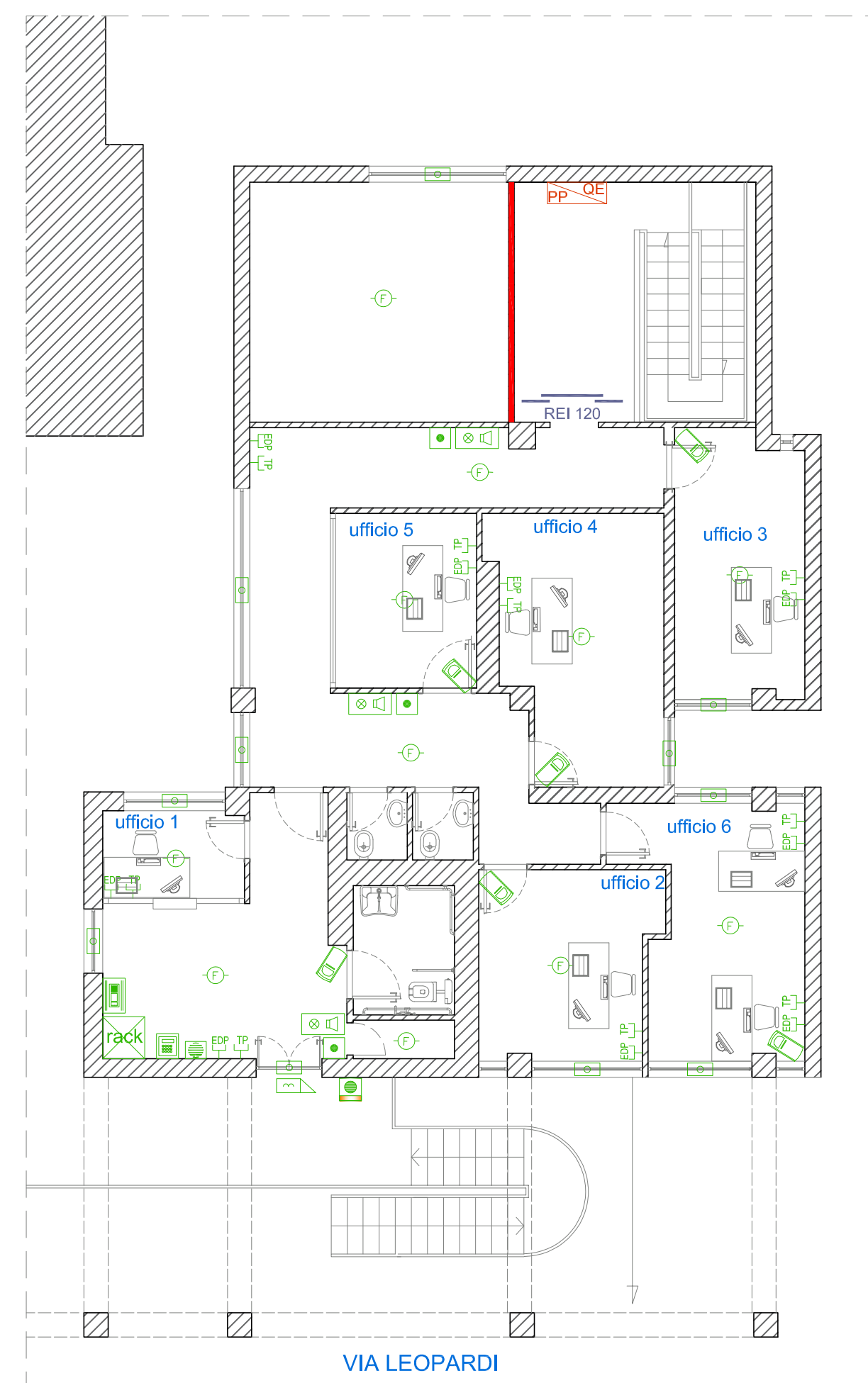
PIANTA PIANO PRIMO UFFICI
