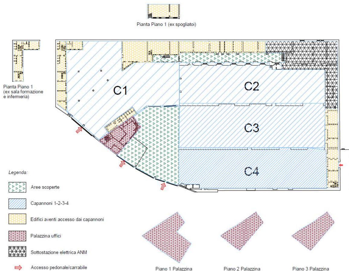
Figura 6 - Schema funzionale di progetto
