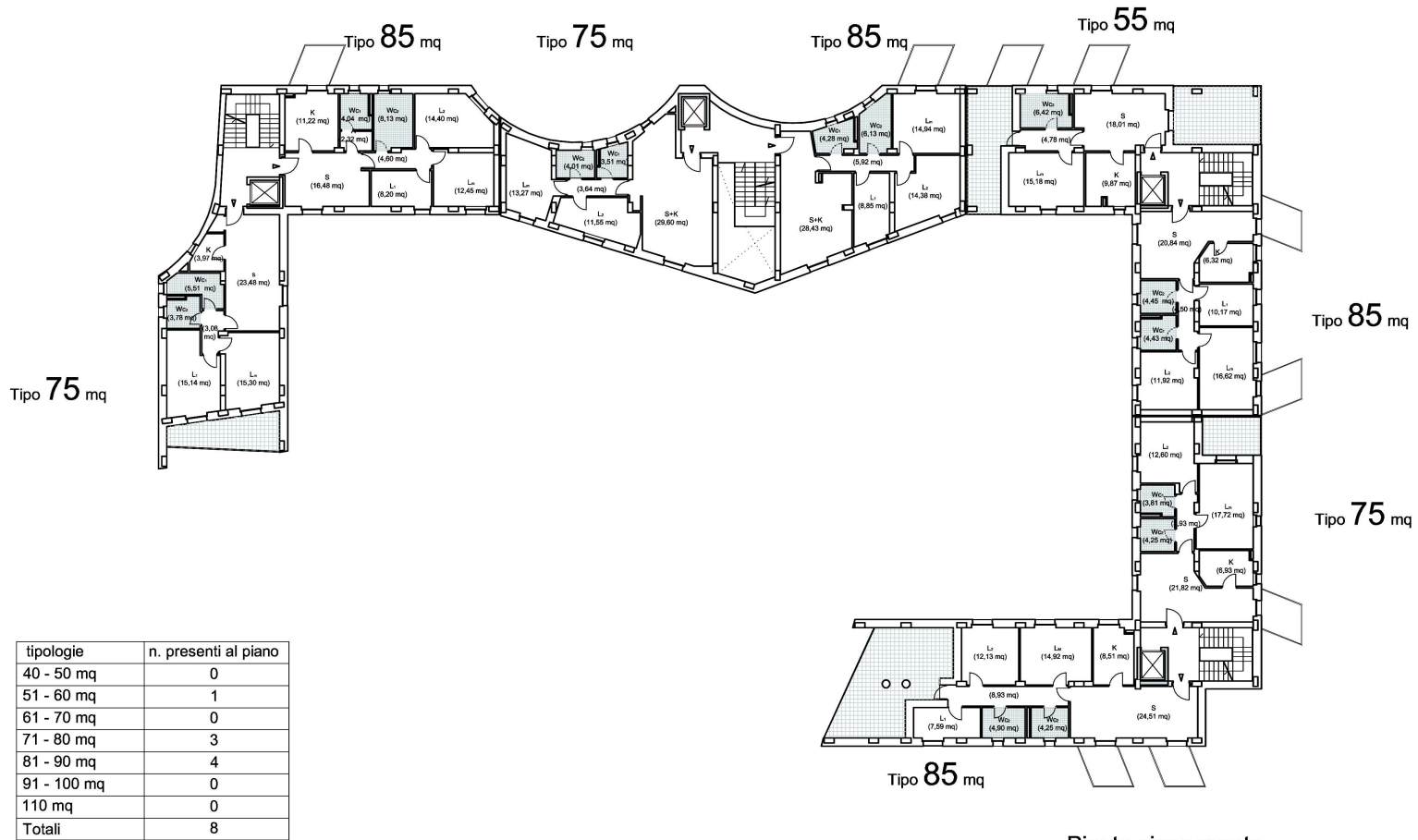
Pianta piano quarto
