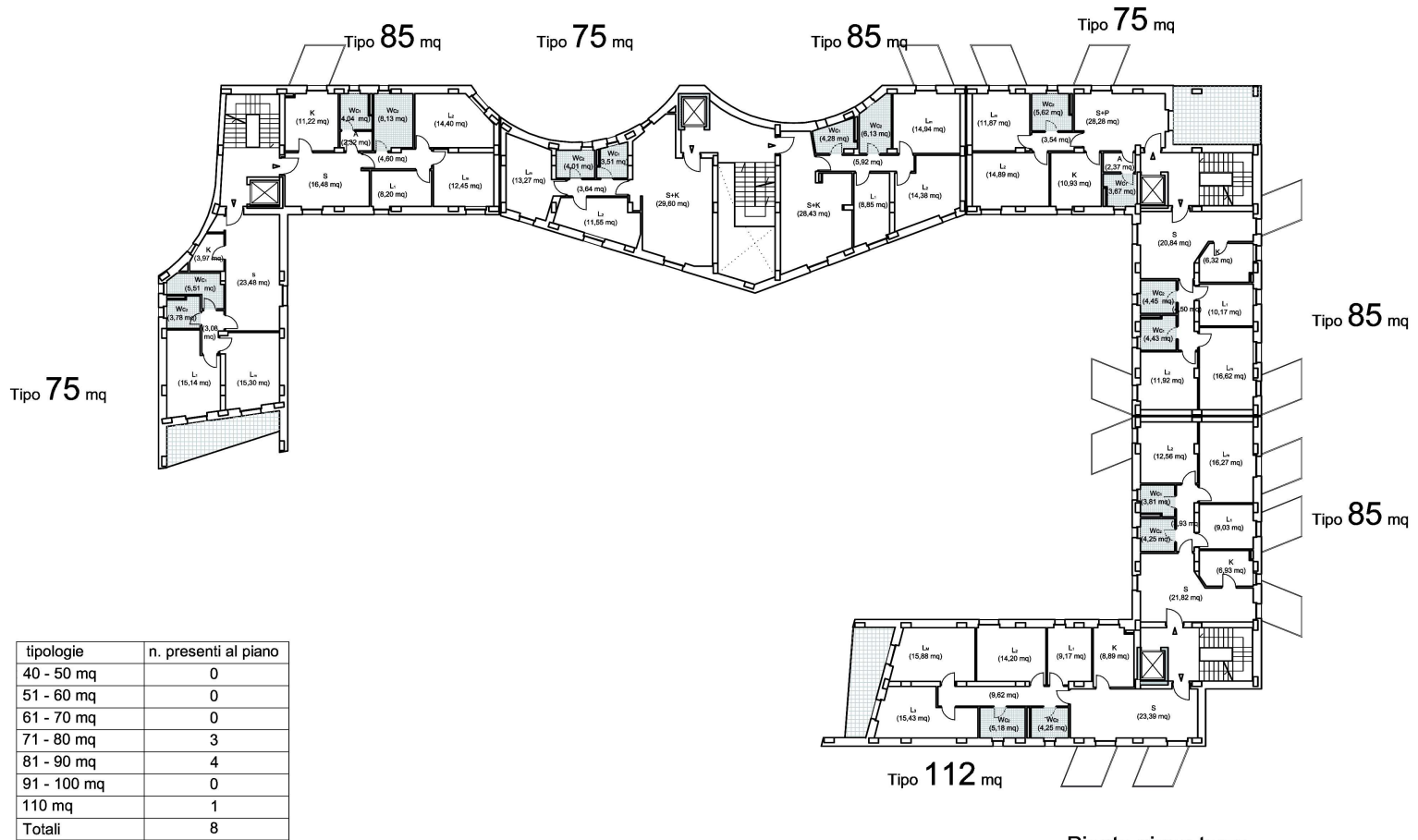
Pianta piano terzo 0 5m N
