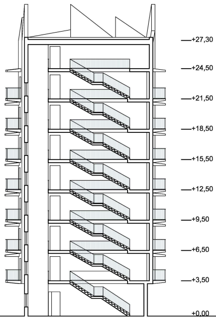
Sezione B - B' Scala 1:200
